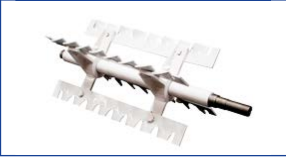
Rotor / Rotor / Rotor à Palette
